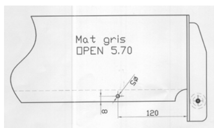
Cotes de perçage vis métaux + écrou
